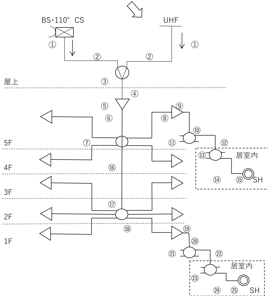
受信システム系統図-2
